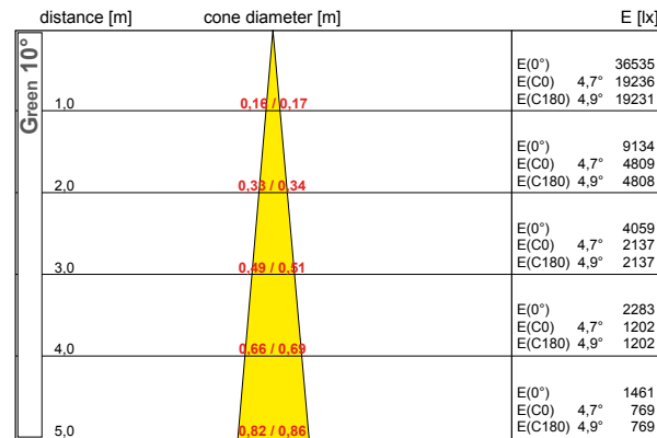
half value angle C0-180 : 9,4° C90-270 : 9,8° 24xLED, total flux: 1680,0 lm, LOR: 95%
