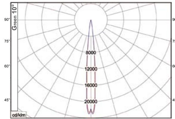
— C0-C180 — C90-C270 half value angle C0-180 : 9,4° C90-270 : 9,8°
