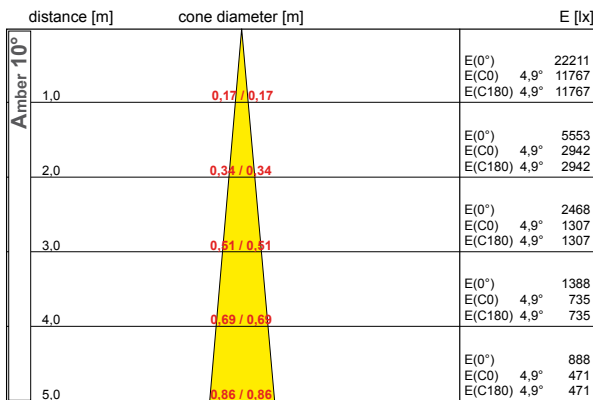
half value angle C0-180 : 9,8° C90-270 : 9,8° 30xLED, total flux: 1440,0 lm, LOR: 68%
