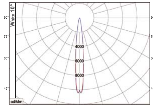
— C0-C180 — C90-C270 half value angle C0-180 : 11,4° C90-270 : 11,8°
