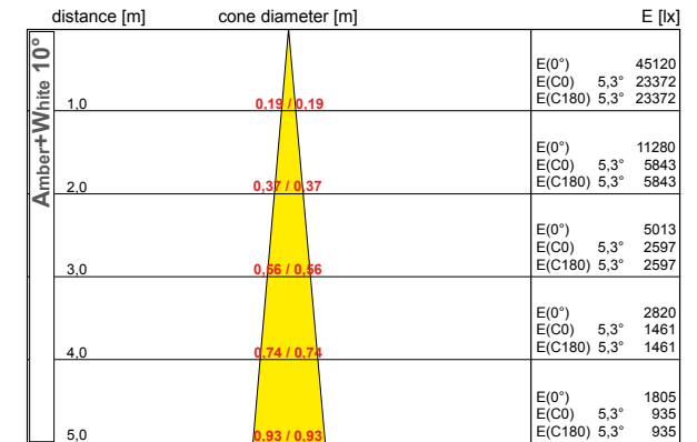
half value angle C0-180 : 10,6° C90-270 : 10,6° 54xLED, total flux: 3840,0 lm, LOR: 69%
