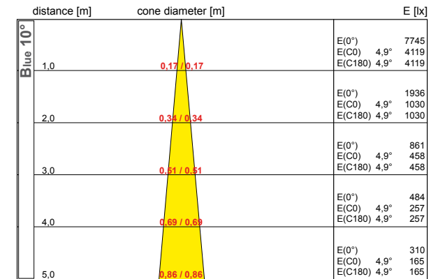
half value angle C0-180 : 9,8° C90-270 : 9,8° 24xLED, total flux: 528,0 lm, LOR: 69%
