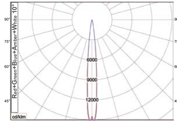
— C0-C180 — C90-C270 half value angle C0-180 : 9,8° C90-270 : 10,2°
