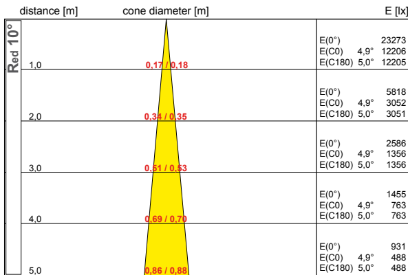
half value angle C0-180 : 9,8° C90-270 : 10,0° 30xLED, total flux: 1440,0 lm, LOR: 78%
