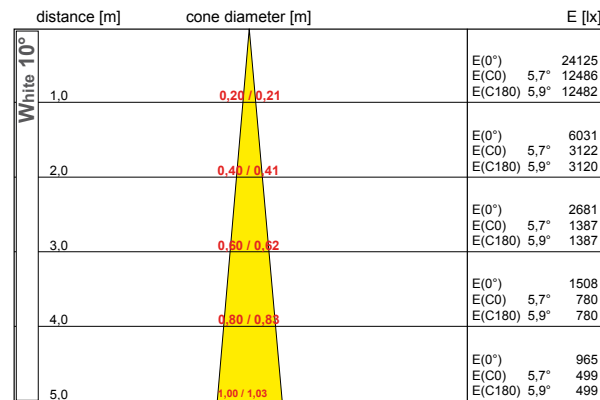
half value angle C0-180 : 11,4° C90-270 : 11,8° 24xLED, total flux: 2400,0 lm, LOR: 71%
