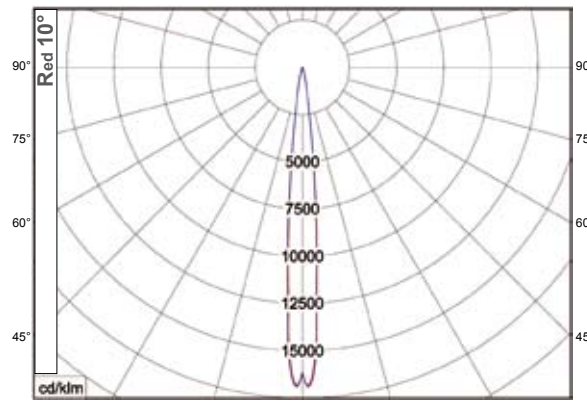
— C0-C180 — C90-C270 half value angle C0-180 : 9,8° C90-270 : 10,0°
