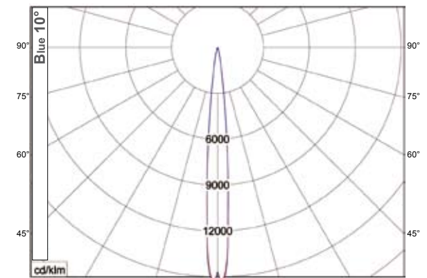
— C0-C180 — C90-C270 half value angle C0-180 : 9,8° C90-270 : 9,8°
