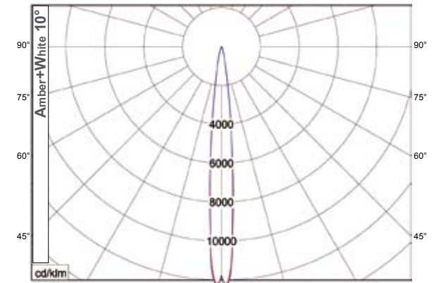
— C0-C180 — C90-C270 half value angle C0-180 : 10,6° C90-270 : 10,6°
