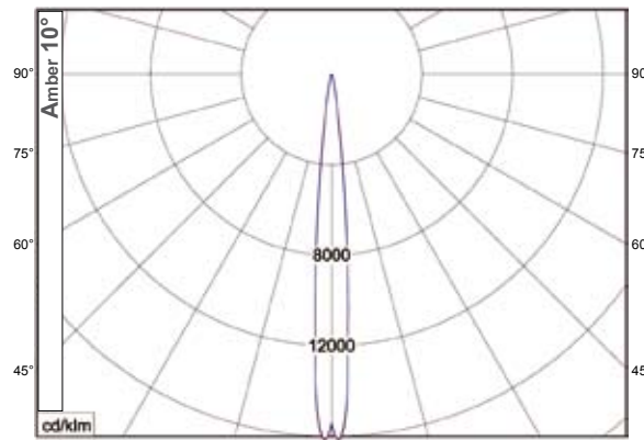
— C0-C180 — C90-C270 half value angle C0-180 : 9,8° C90-270 : 9,8°
